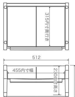
エコボックス単体
