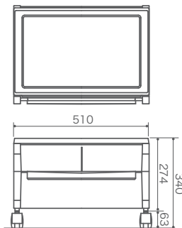
エコボックス 天板・キャスター付
