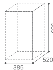
エコボックス単体 梱包単位 / 3 荷姿 / ダンボール 梱包重量 / 6.8kg 梱包サイズ / W385×D520×H585
