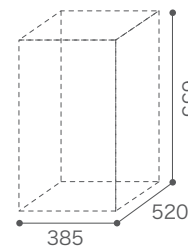
エコボックス 天板・キャスター付 梱包単位 / 3 荷姿 / ダンボール 梱包重量 / 10.5kg 梱包サイズ / W385×D520×H655
